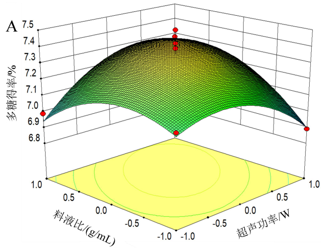
图2 各试验因素交互作用的响应面和等高线图
